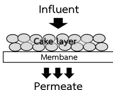
ภาพที่ 2.4 ไมโครฟิลเตรชันแบบ Dead-End (Dead-End Microfiltration)
