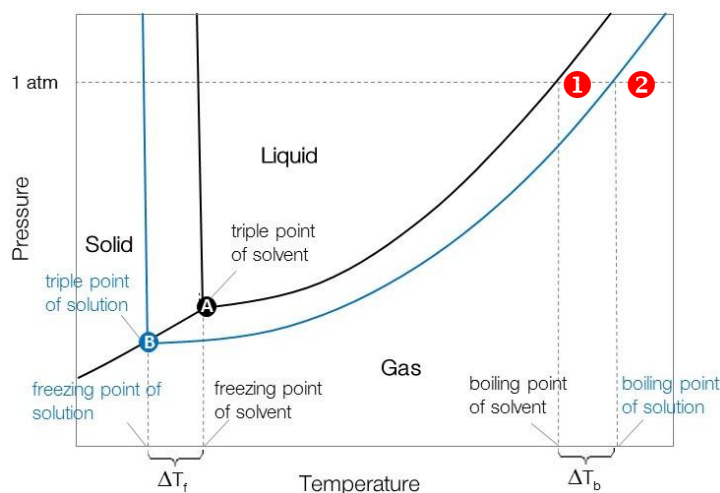
ภาพที่ 2.5 วัฏภาคแสดงการเปลี่ยนแปลงของจุดเยือกแข็งและจุดเดือดของสารบริสุทธิ์และสารละลาย. ดัดแปลงจาก Chemistry: The Central Science (p.545-546), by T.L. Brown et al., 2017
