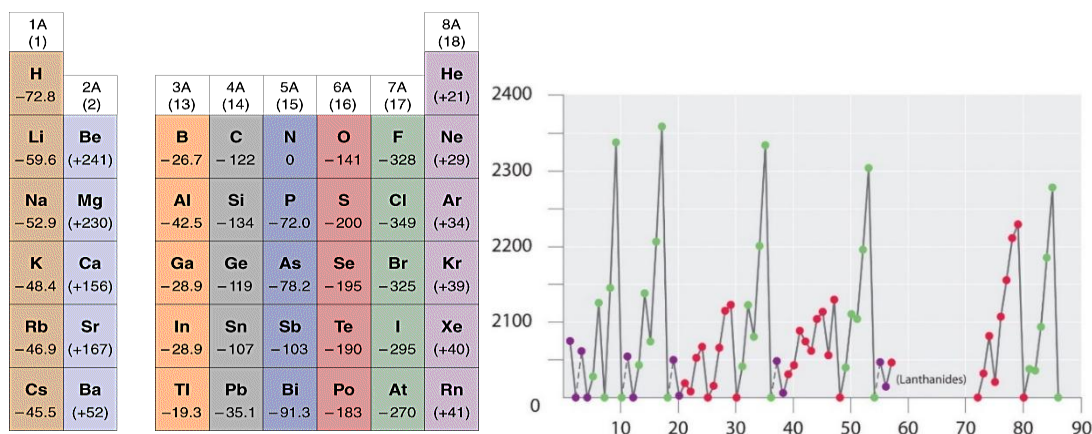
ภาพที่ 1.11 ค่าสัมพรรคภาพอิเล็กตรอนของธาตุเรพรีเซนเททีฟ ที่มา: Silberberg. Principle of General Chemistry. 2013. p264
