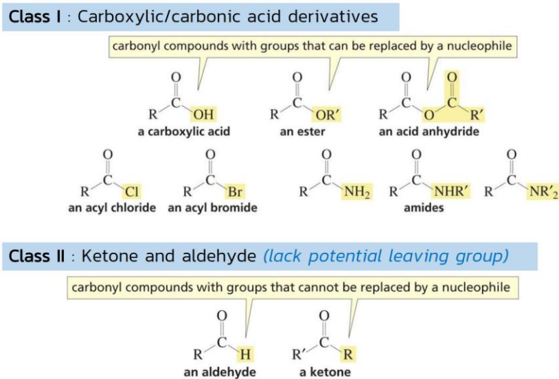
ภาพที่ 6.10 กลุ่มของสารประกอบคาร์บอนิล
