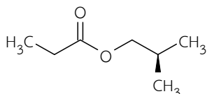
isobutyl propionate (rum)
