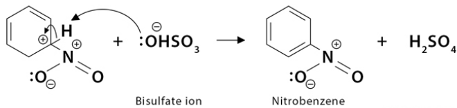
ภาพที่ 8.9 กลไกปฏิกิริยาไนเตรชัน
