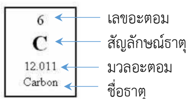
ภาพที่ 1.1 สัญลักษณ์นิวเคลียร์ของธาตุคาร์บอน
