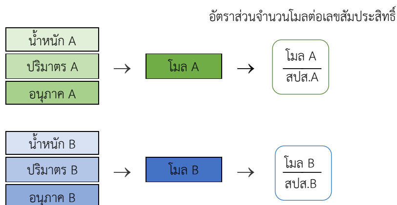
ภาพที่ 1.16 แนวคิดการหาสารกำหนดปริมาณในกรณีที่สารตั้งต้นมีสัมประสิทธิ์จำนวนโมลไม่เท่ากัน
