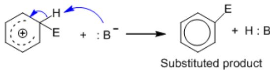
ภาพที่ 5.12 กลไกปฏิกิริยาการแทนที่ด้วยอิเล็กโตรไฟล์
