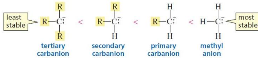
ภาพที่ 5.4 ประเภทและลำดับความเสถียรของคาร์แบนไอออน
