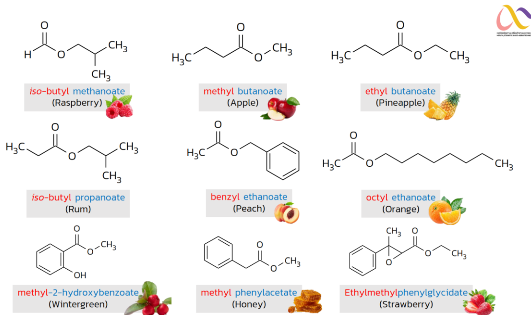
ภาพที่ 4.17 เอสเทอร์ที่พบในธรรมชาติ
