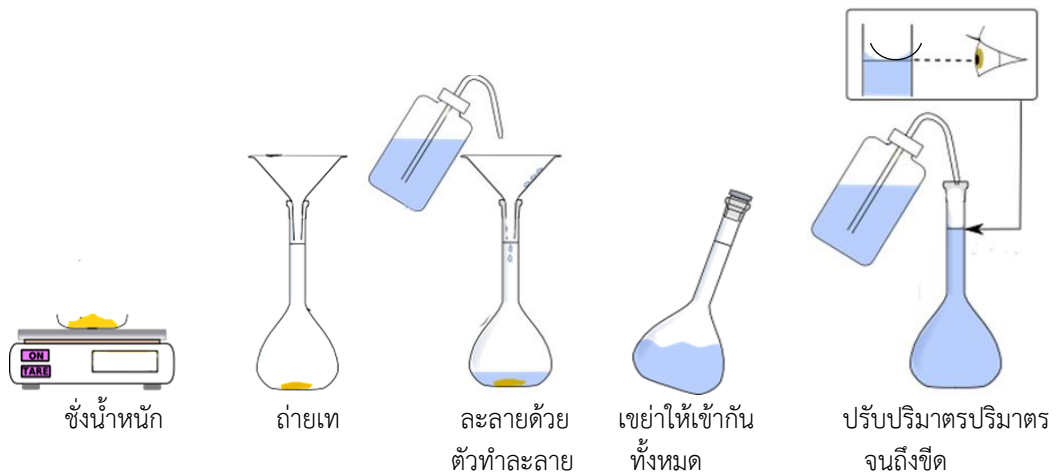
ภาพที่ 2.11 ขั้นตอนการเตรียมสารละลายจากสารสถานะของแข็ง. จาก เคมีวิเคราะห์: หลักการและเทคนิคการคำนวณเชิงปริมาณ (หน้า 43) โดย วรวิทย์ จันทร์สุวรรณ, 2565, สำนักพิมพ์จุฬาลงกรณ์มหาวิทยาลัย.
