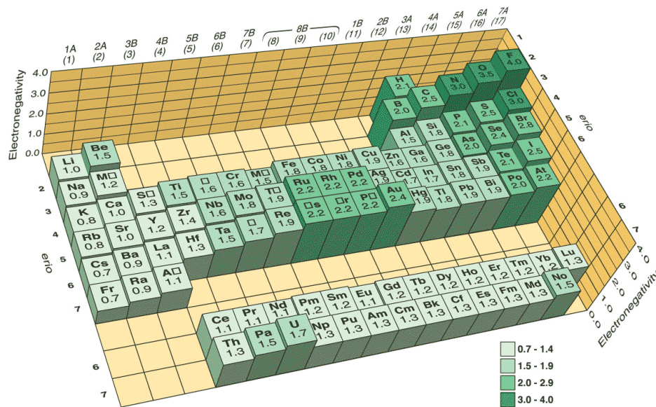
ภาพที่ 1.12 แนวโน้มค่าอิเล็กโทรเนกาติวิตีของพอลิง
