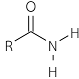
สูตรทั่วไปของเอไมด์
