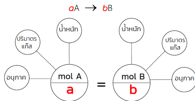
ภาพที่ 1.14 แนวคิดการคำนวณปริมาณสัมพันธ์โดยวิธีโมลสัมพันธ์
