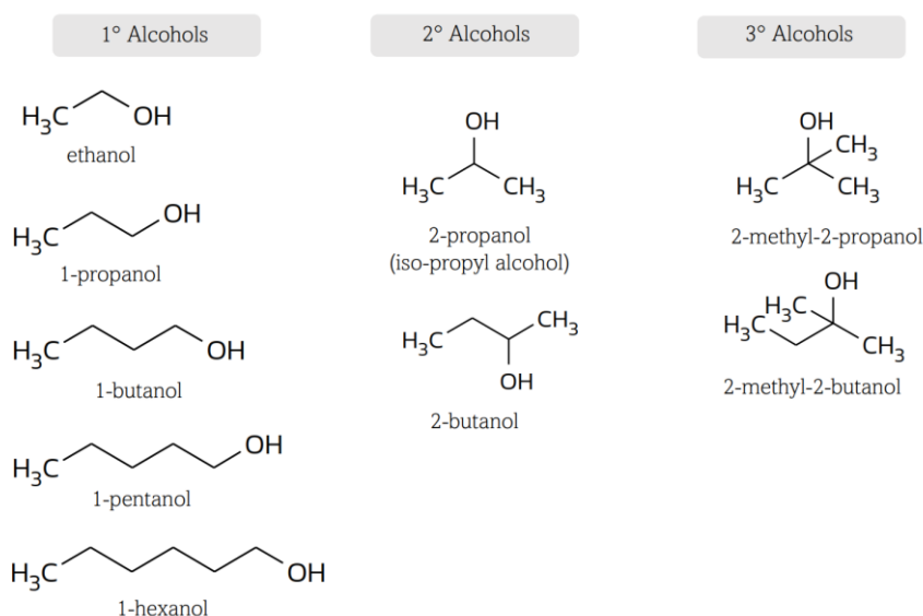
ภาพที่ 6.2 โมโนไฮดริคแอลกอฮอล์
