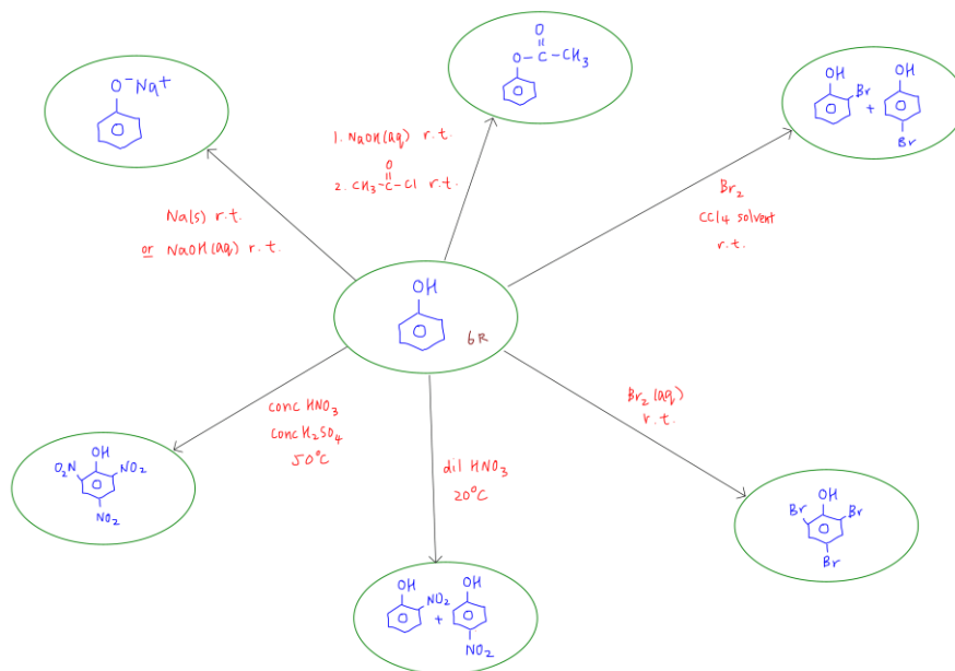
ภาพที่ 6.7 แผนผังปฏิกิริยาฟีนอล ( https://chemistryguru.com.sg/alcohol-reactions-organic-chemistry )
