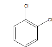
1,2-dichlorobenzene
