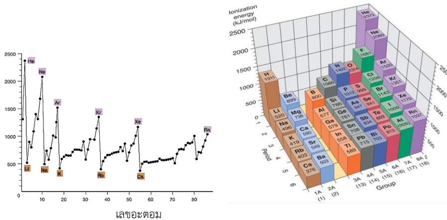
ภาพที่ 1.10 แนวโน้มพลังงานไอออไนเซชันลำดับที่ 1
